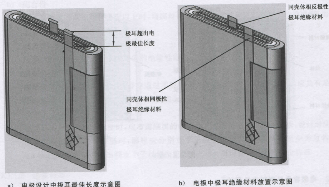
图 B.3 电极中极耳布局
