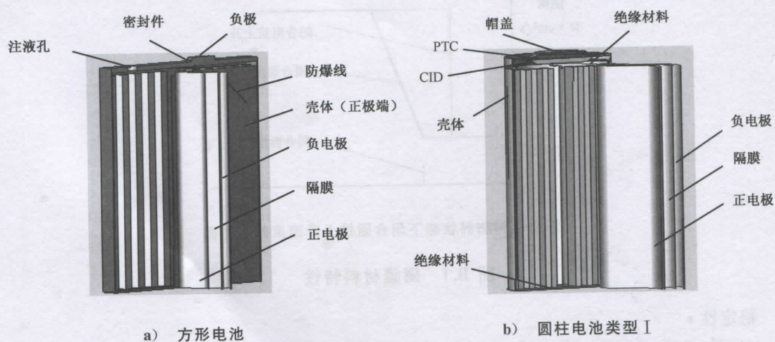
图 B.2 锂离子电池结构实例
