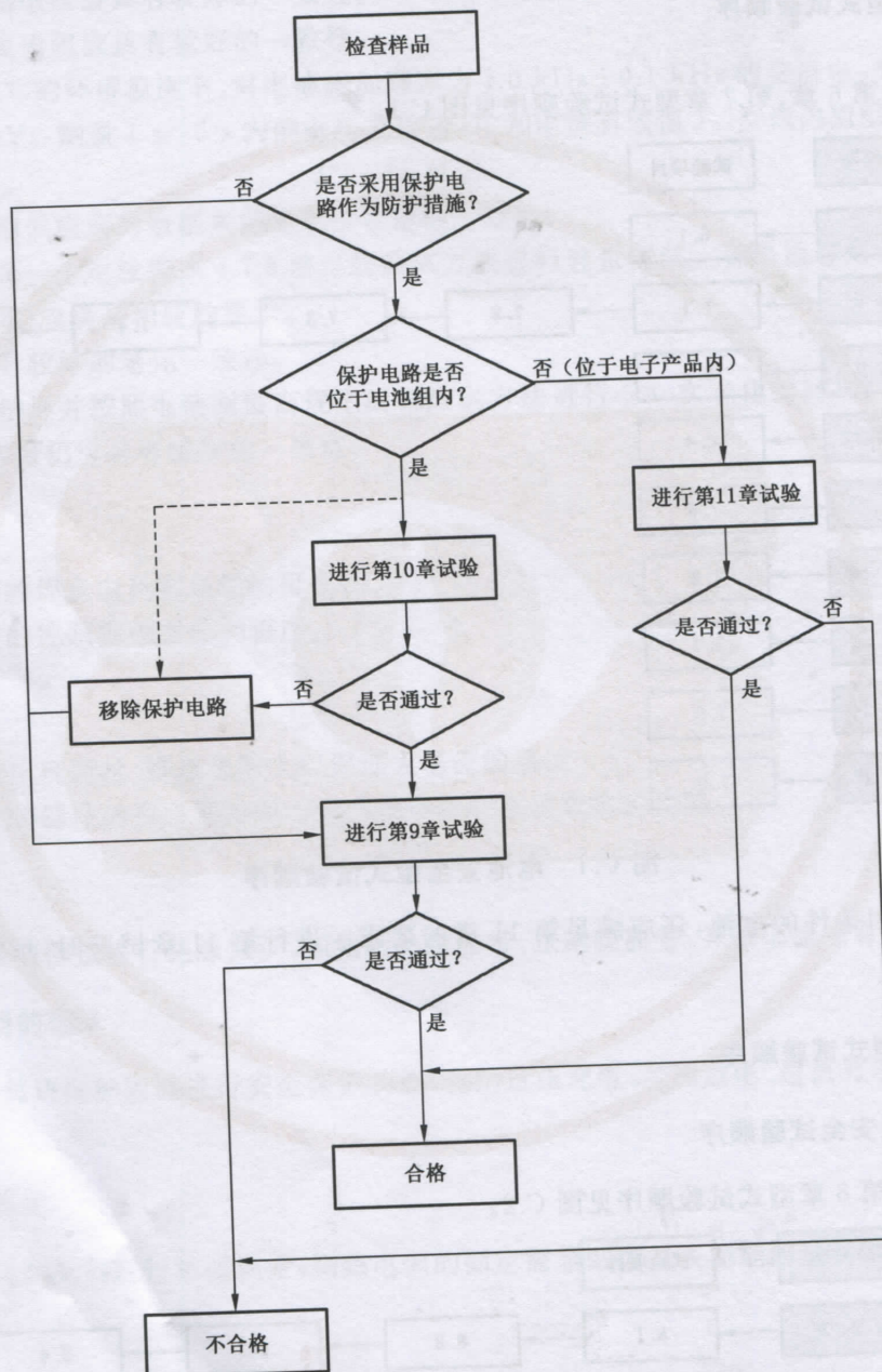
图 C.3 电池组电安全试验顺序
