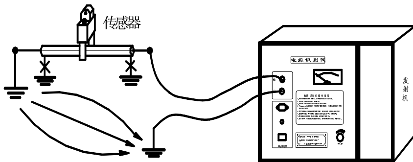
图 2 识别仪接线图
