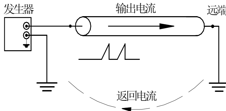
图 3 基本电路
