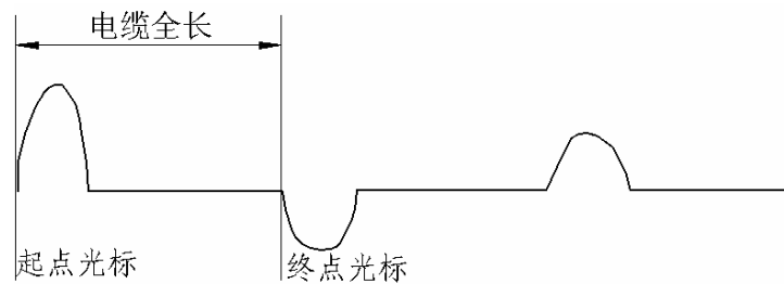
图 8.4 闪络测试故障点不放电波形
