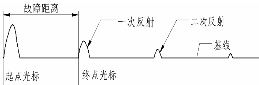
图 8.1 低压脉冲测全长波形
