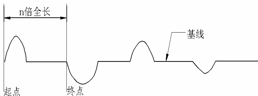
图 8.6 近端故障冲闪测试波形
