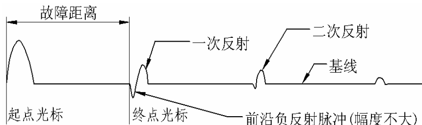
图 8.3 闪络法电流取样测试波形
