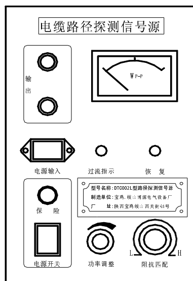
图 4.1 路径仪面板示意图
