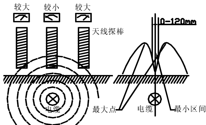
图 9.1 电缆周围磁场分布及路径探测原理示意图
