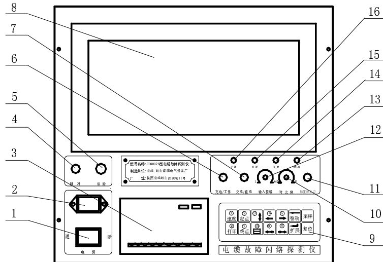
图 2.1 闪测仪面板示意图
