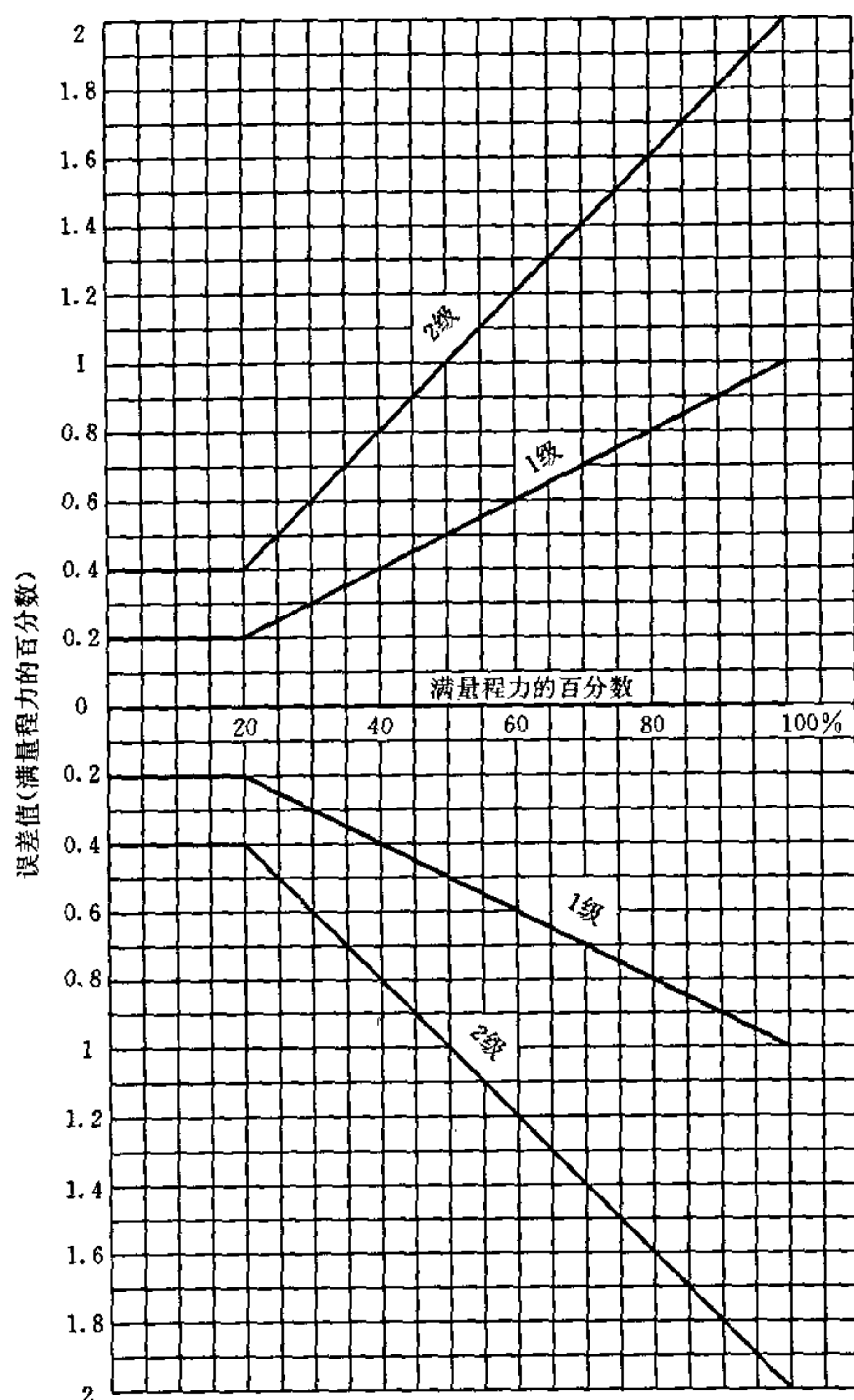
图 1 试验机的分级
