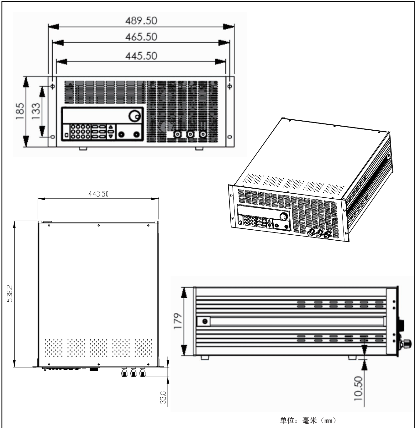
▼ IT6160系列电源尺寸图
