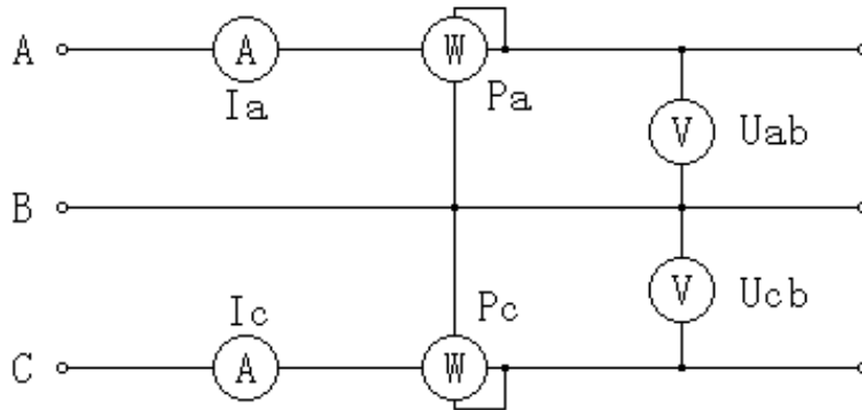
图二十、三相三线计量原理图
