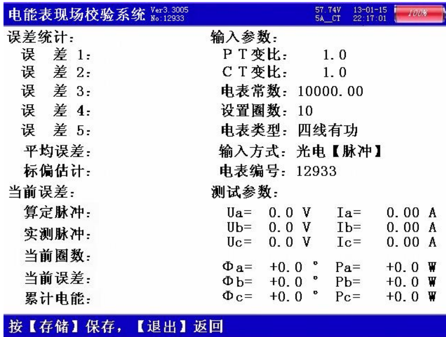
图七、电表校验屏
