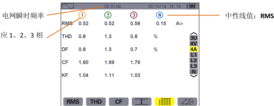
图 8-18 4A 下各值同时显示屏幕
