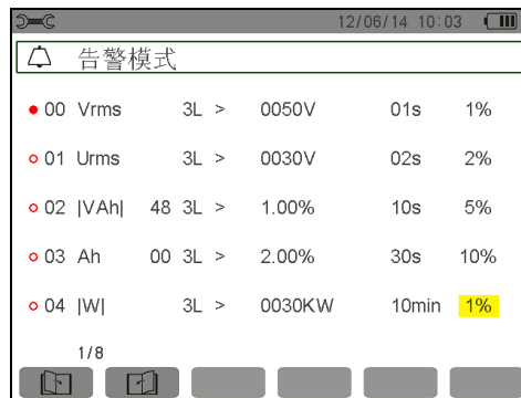
图 5-15 告警模式菜单
