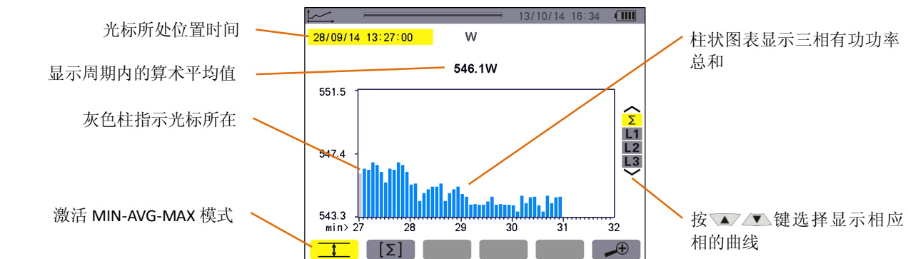
图 10-15 三相有功功率总和包括最大、最小、平均值
