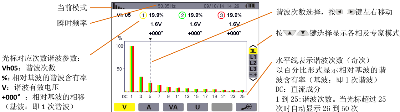
图 7-2 相电压谐波 3L 显示
