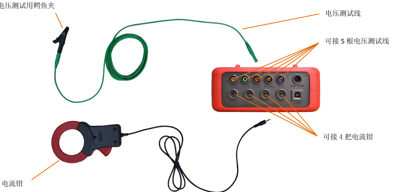
图 4-3 顶端测试连接
