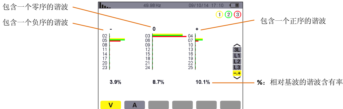
图 7-10 相电压的专家模式显示
