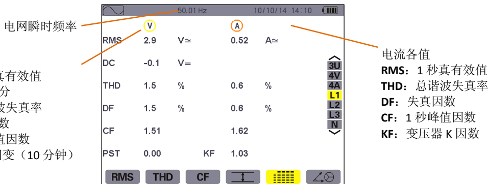
图 8-19 L1 下各值同时显示屏幕
