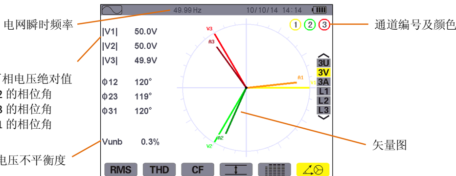
图 8-20 3V 下矢量图显示屏幕
