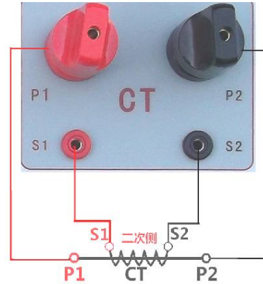
图 13, CT 变比极性接线图
