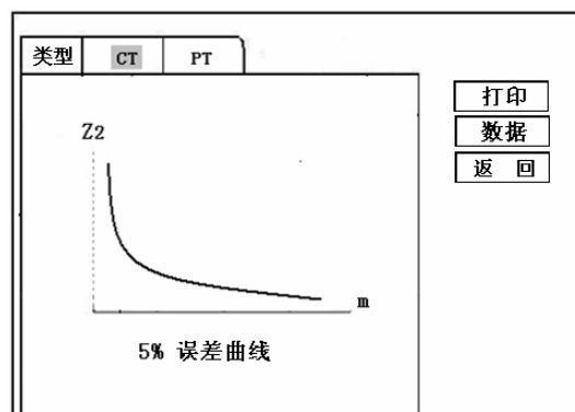
图 9, 误差曲线图
