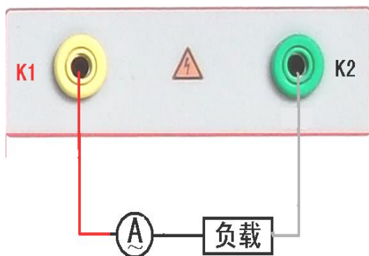
图 37，电流校准接线图
