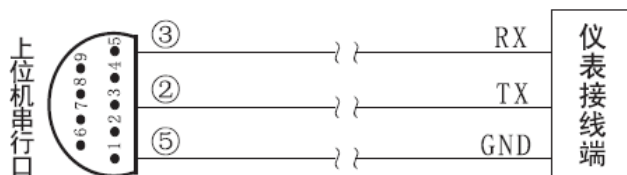
RS-232 通讯
