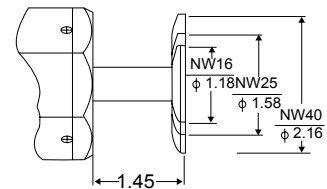
ISO NW 真空接头
