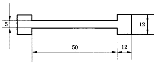
图 3 哑铃试样
