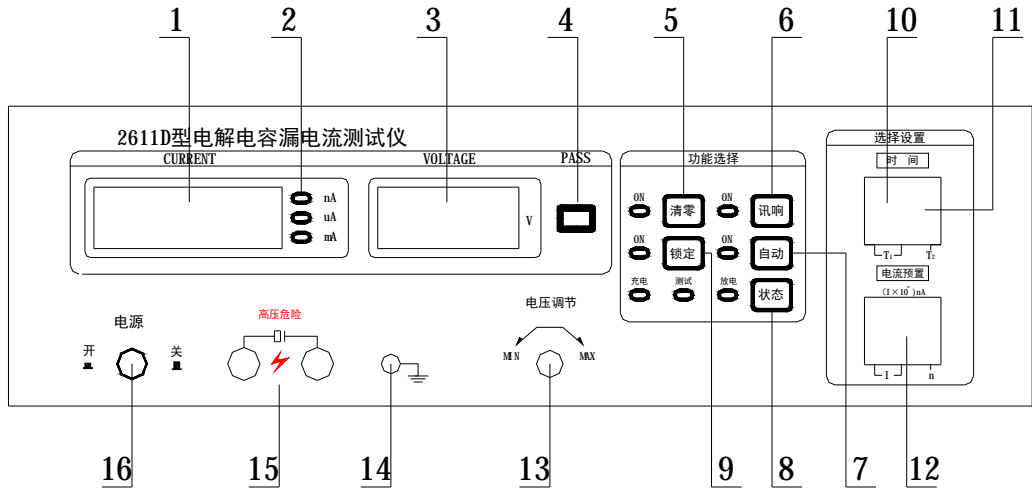
图 3-3 前面板
