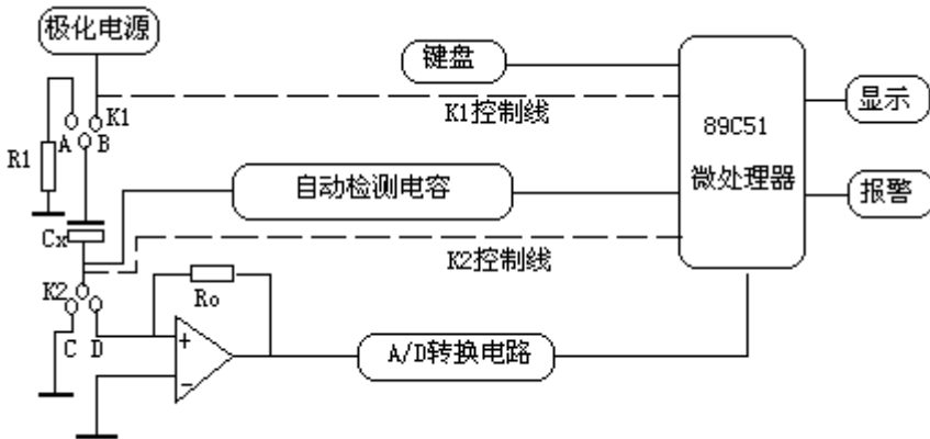
图 3-2 框图
