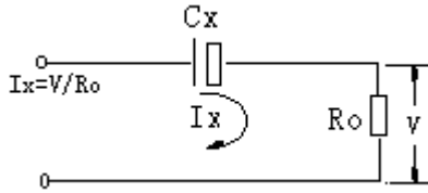
图 3-1 测试原理
