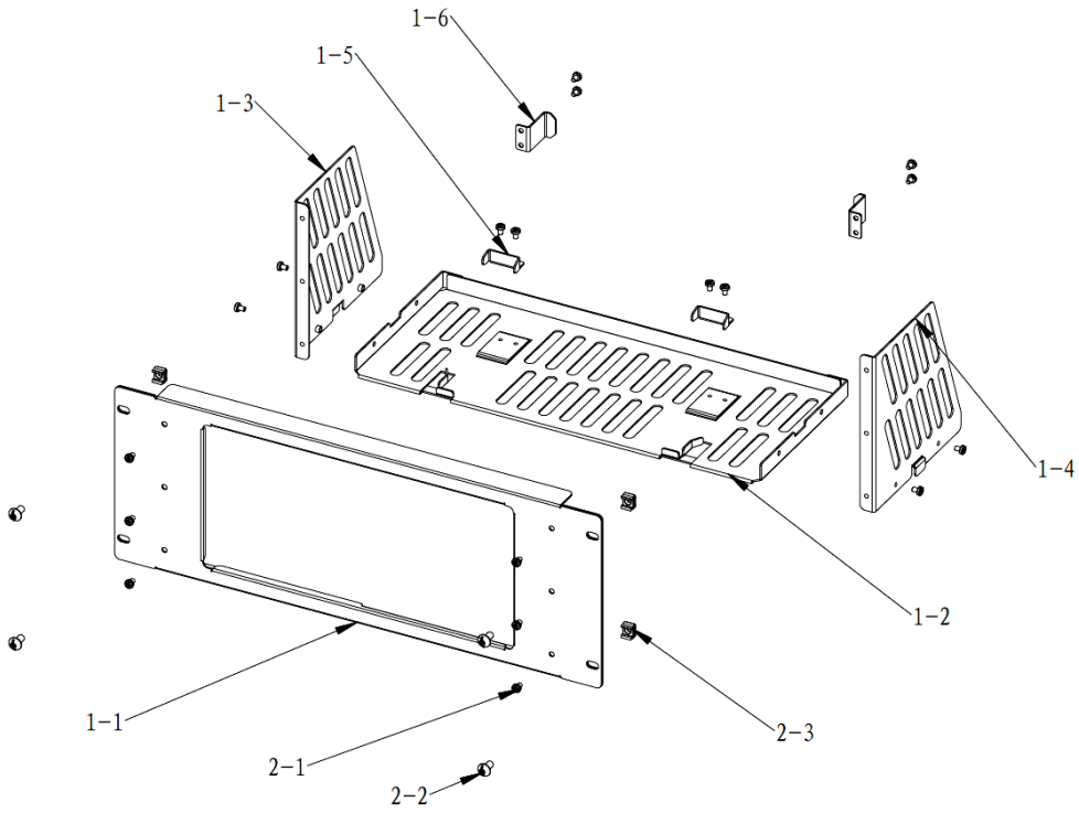
图 1-11 机架部件
