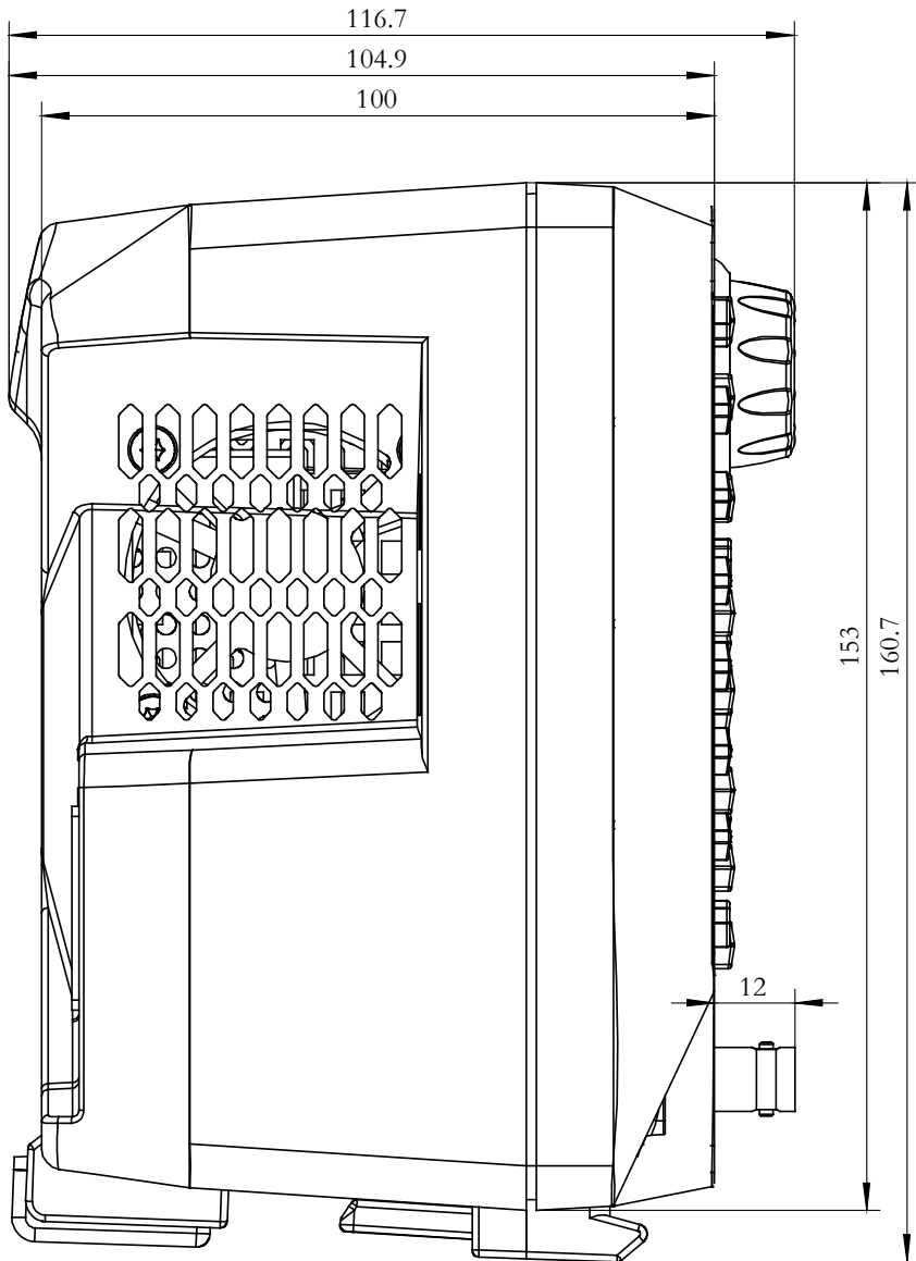
图 1-4 侧视图
