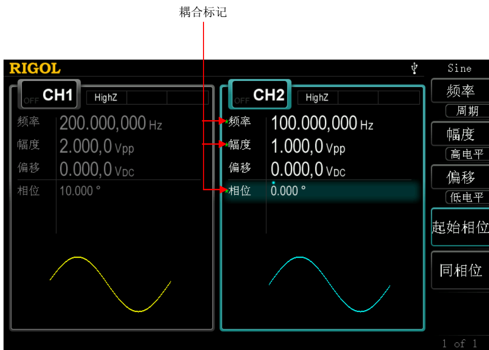
图 10-4 通道耦合
