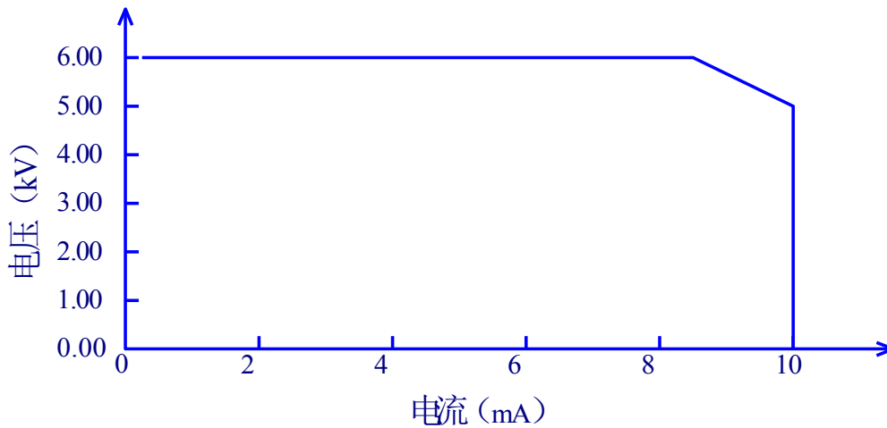
图 3-4 JK9310 直流电压输出范围
