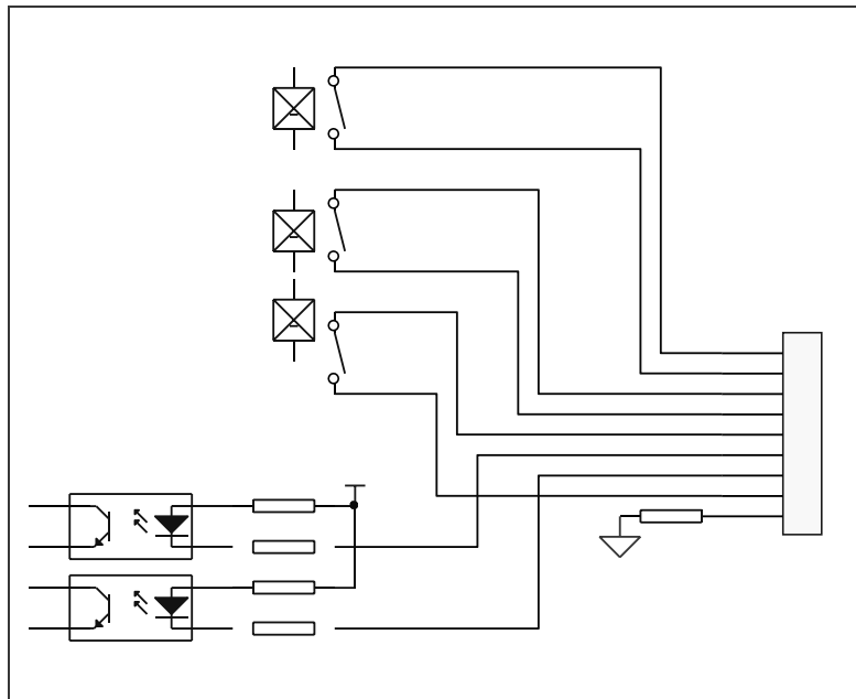
仪器内部 HANDLER 电路连接示意图
