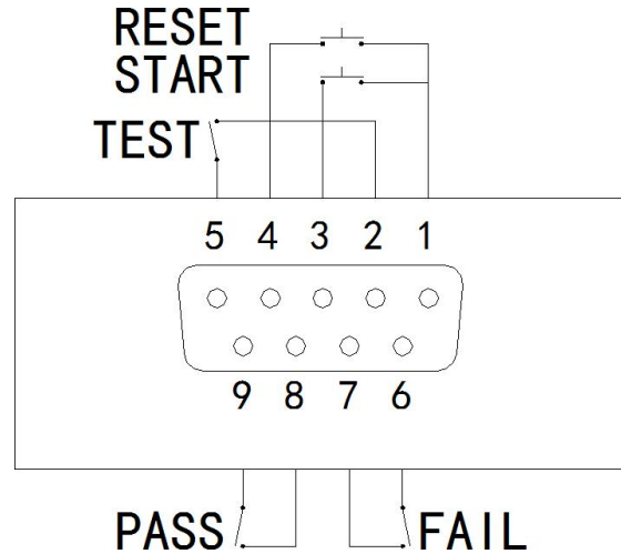
HANDLER 外部电路连接示意图
