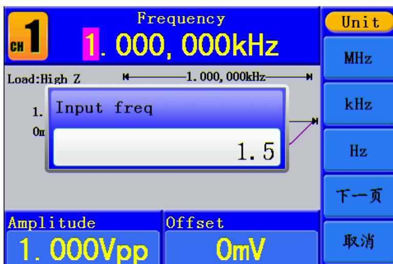
图 5-3: 使用数字键盘设置频率
