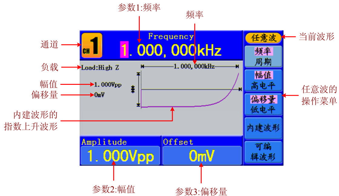
图 5-11：任意波用户界面
