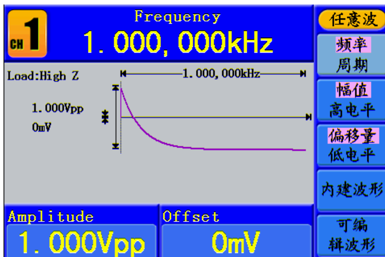
图 5-12: 指数下降内建波形
