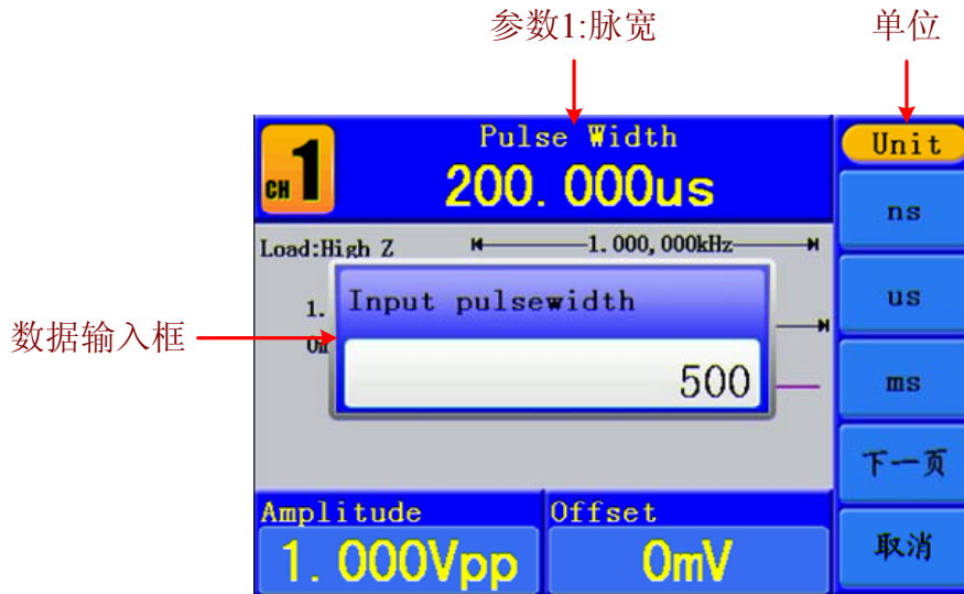
图 5-9: 设置脉冲波的脉宽
