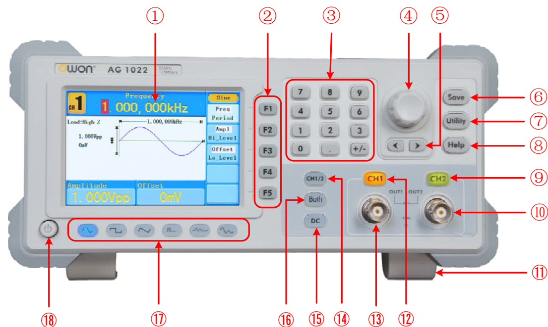
图 4-1 前面板概览
