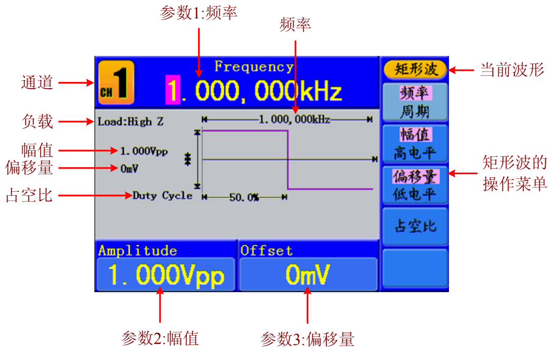
图 5-4: 矩形波用户界面
