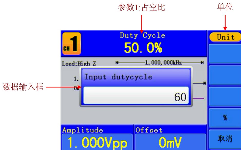
图 5-5: 设置矩形波的占空比
