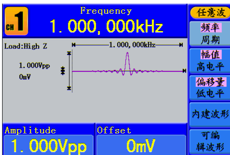
图 5-13: Sin(x)/x 内建波形
