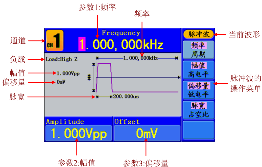
图 5-8: 脉冲波用户界面
