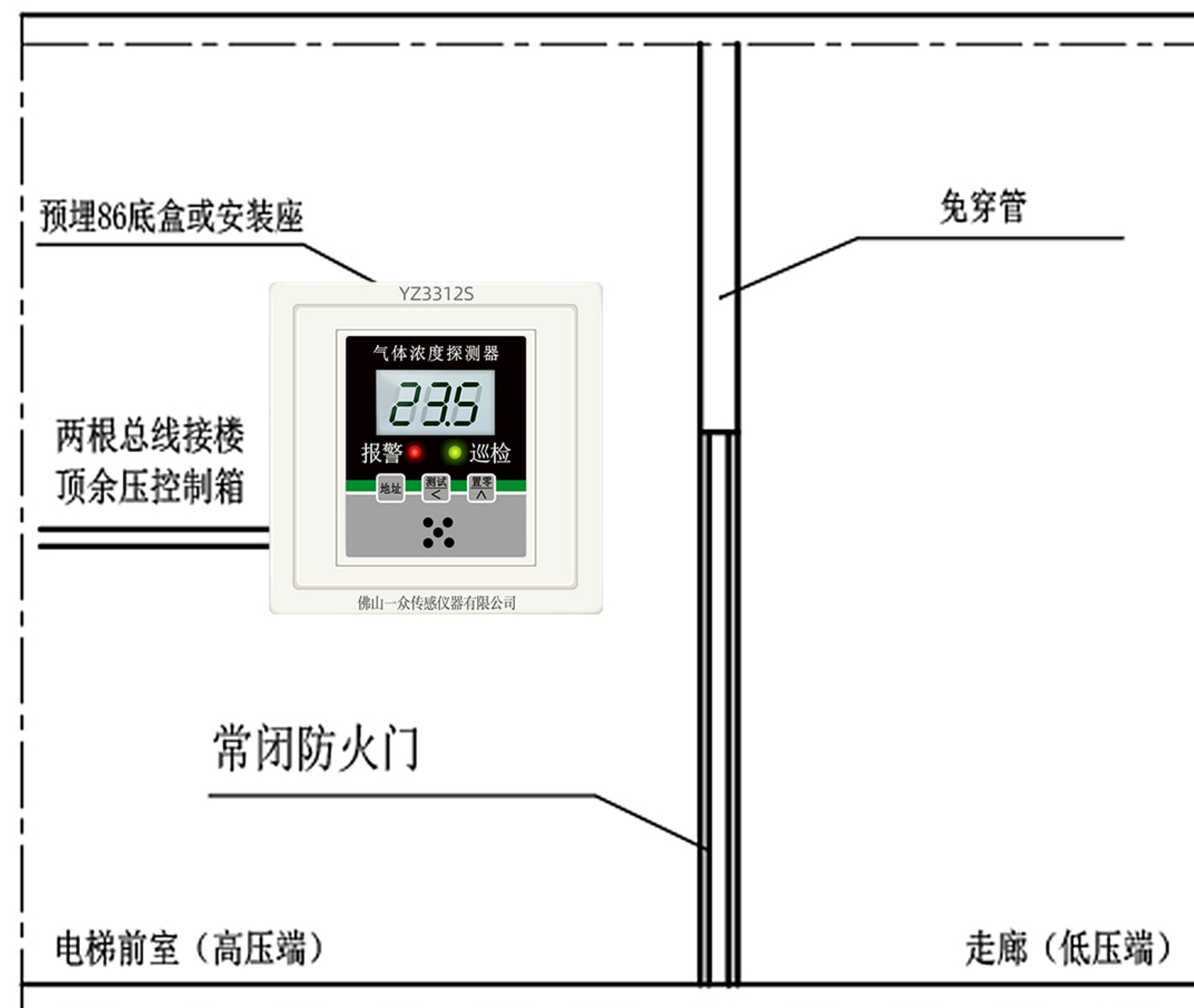
气体浓度探测器安装示意图
