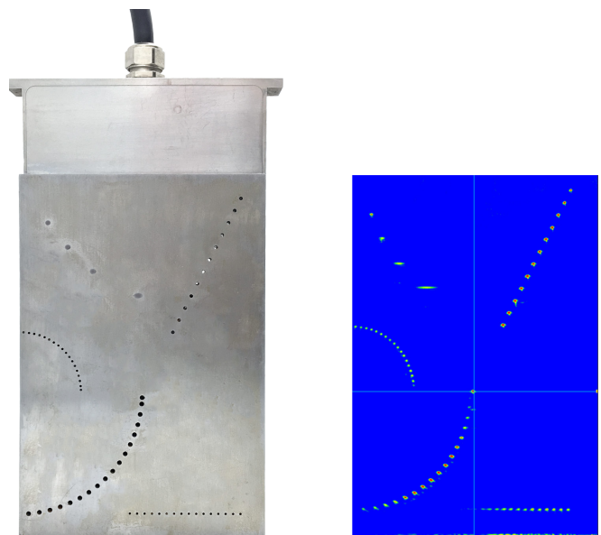
实时全聚焦分辨率可达150万像素
