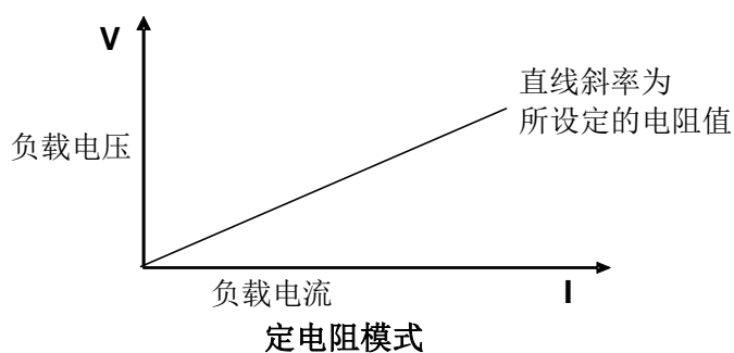
图 3-5 CR 模式电压电流关系图
