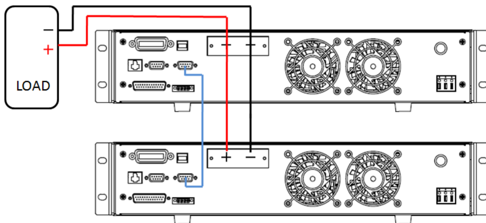
图 2 两台并联的电源设备示意图
