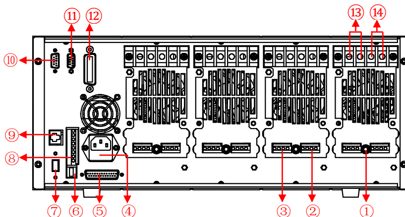
图 2-2 IT8700 后面板图
