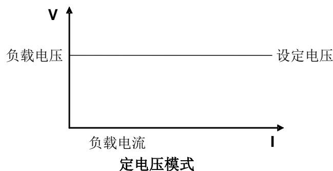
图 4-3 定电压模式电压电流图
