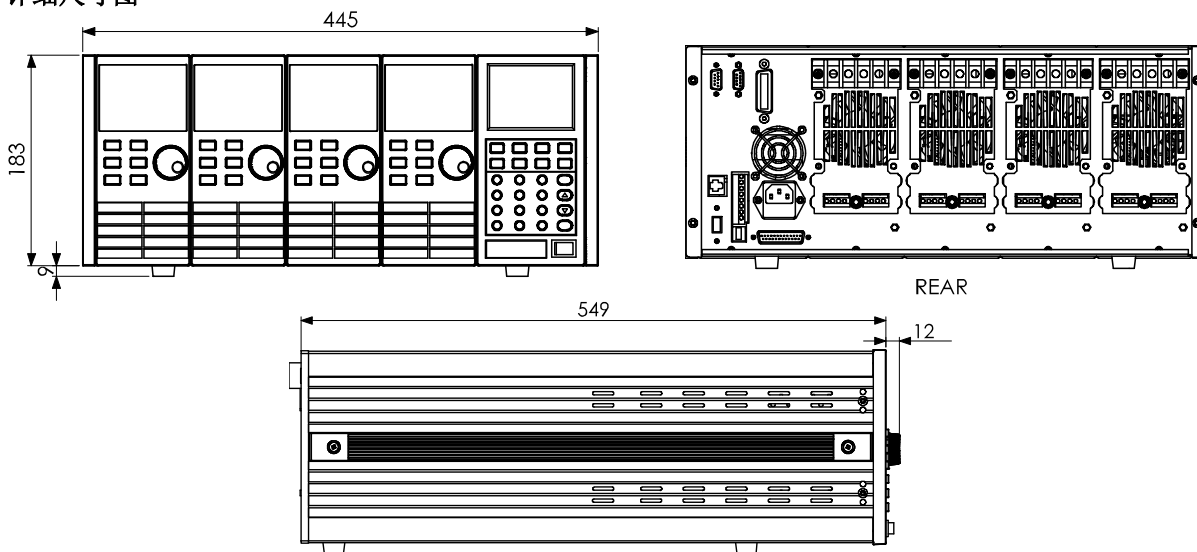
详细尺寸图
