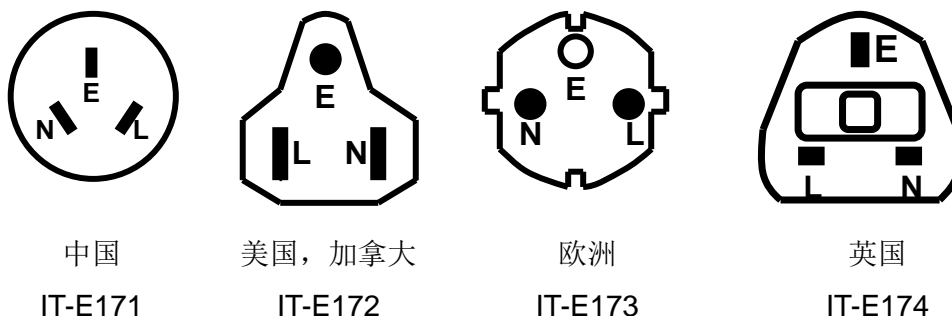
图 1-5 四种电源线型号 (L: 火线 N: 零线 E: 地线)
