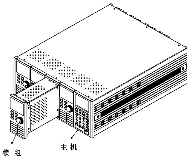
图 1-1 模组安装图
