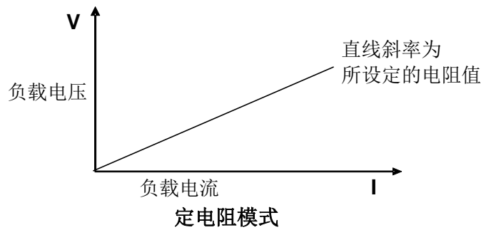
图 4-2 CR 模式电压电流关系图
