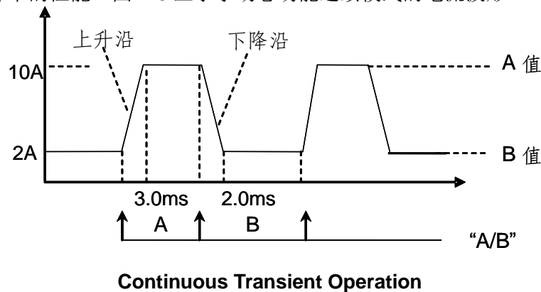
图 4-6 连续模式电流波形
