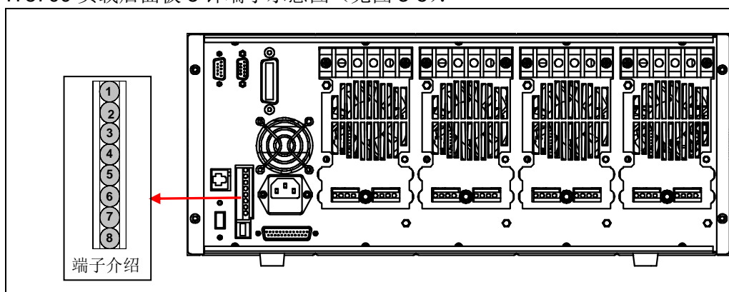
图 3-5 IT8700 后背板 8 针端子
