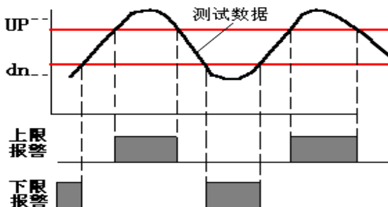
图 3 越限报警判定
