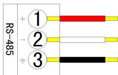
图 4 接线端子示意图
