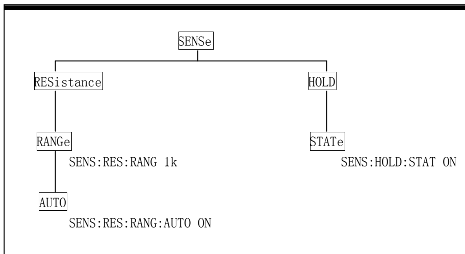
图 6-1 命令树例子
