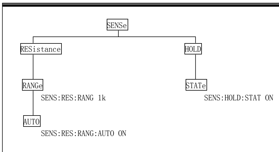
图 6-1 命令树例子
