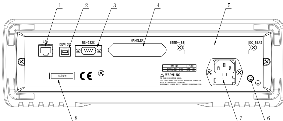
图 2-2. 后面板说明
