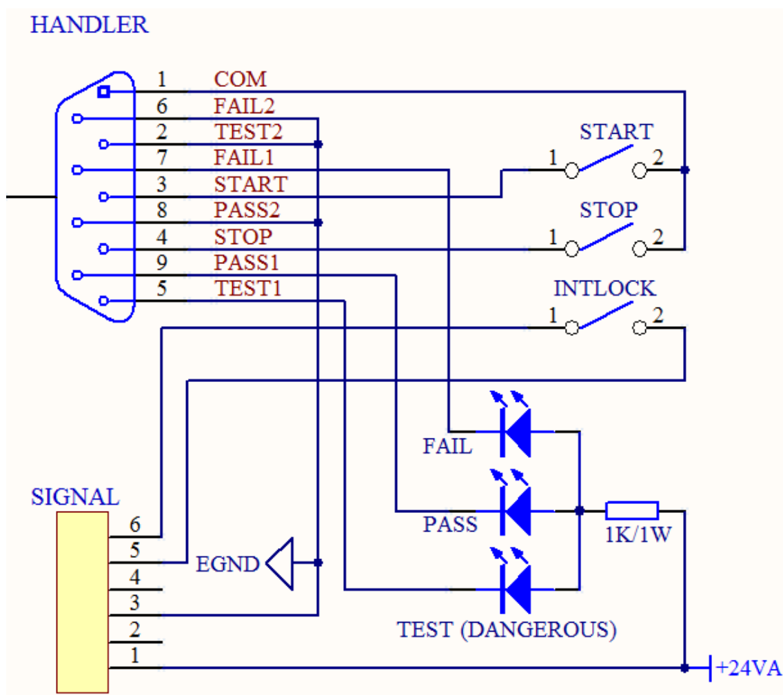
图 4.5.2: 外部电路连接示意图
