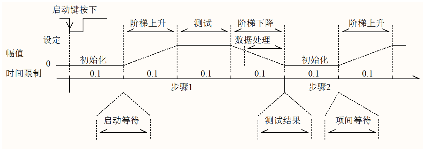
仪器测试时序示意图
