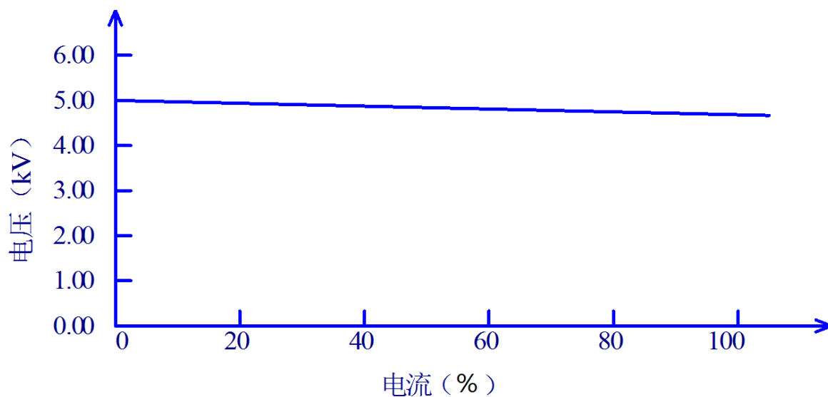
图 3-3 交流电压负载调整率
