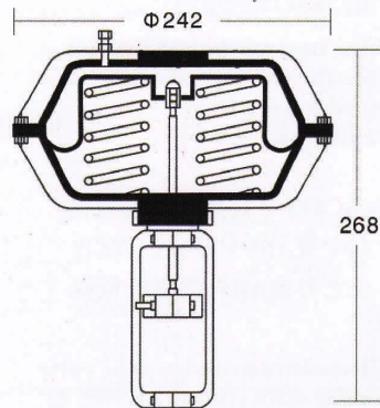
氣動執行器 baelz-P21 Pneumatic Actuator baelz-P21
