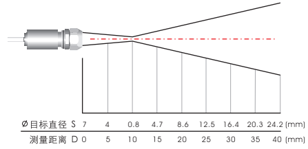
15:1带CF透镜(远距离=1.5:1)
