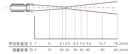
15:1带CF透镜(远距离=1.5:1)
