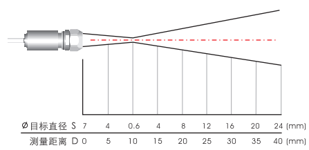
22:1带CF透镜(远距离=1.5:1)
