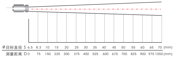
15:1探头
