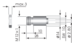
探头
