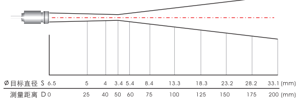
Optics CT LT CF, D:S=15:1 (远距离=5:1)
