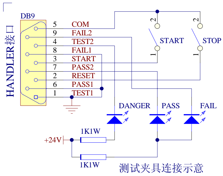
图 4.5.3: HANDLER 外部电路连接示意图
