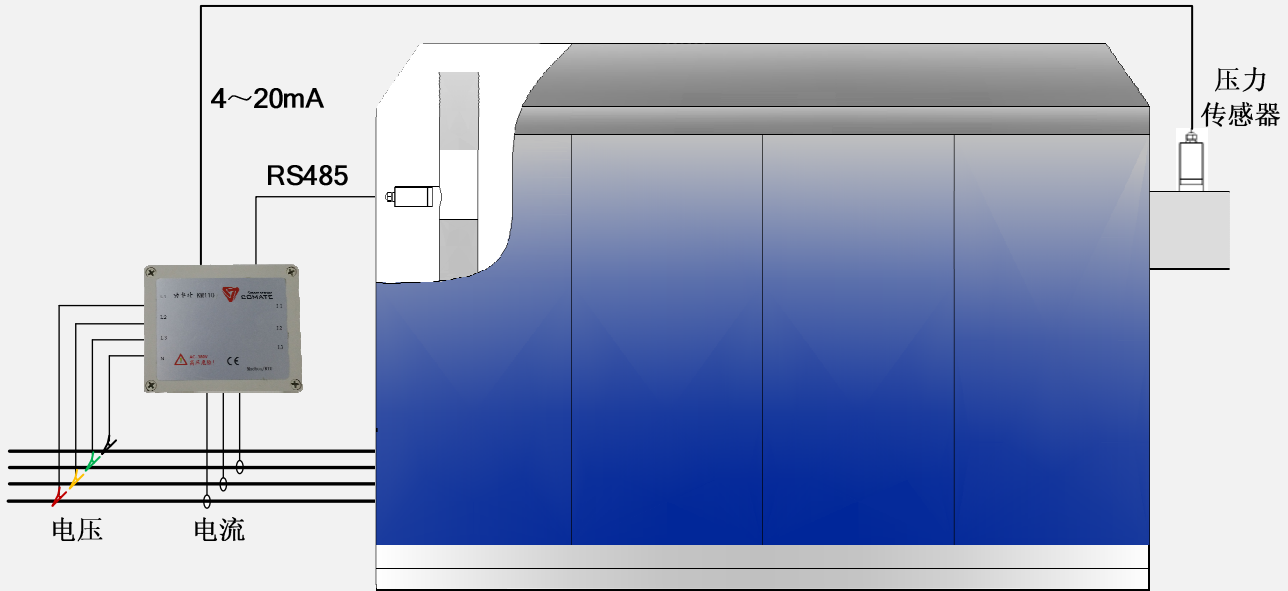
单台空压机接线图
