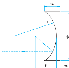
外形图
