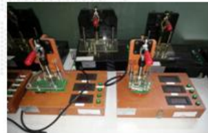
电路测试台
