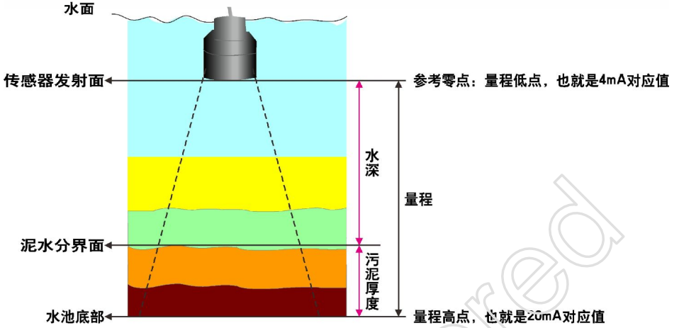
附图 1.1 水深测量示意图
