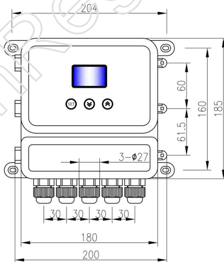
超声波淤泥界面仪结构图
