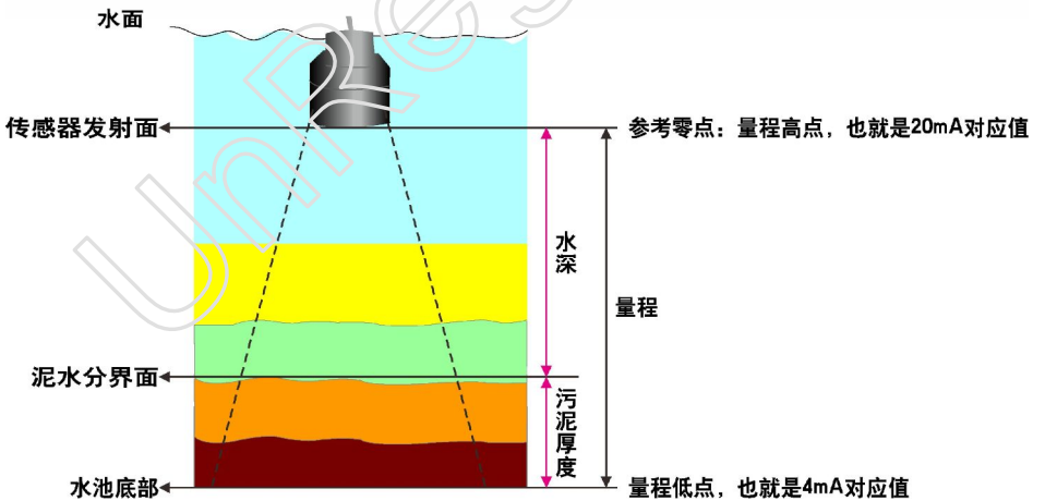
附图 1.2 泥位测量示意图
