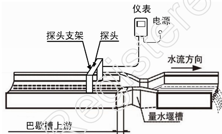
图 7.2.3 巴歇尔槽安装
