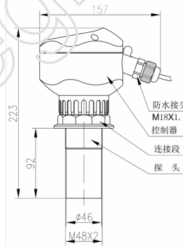
图 4.1.4 明渠流量计结构图
