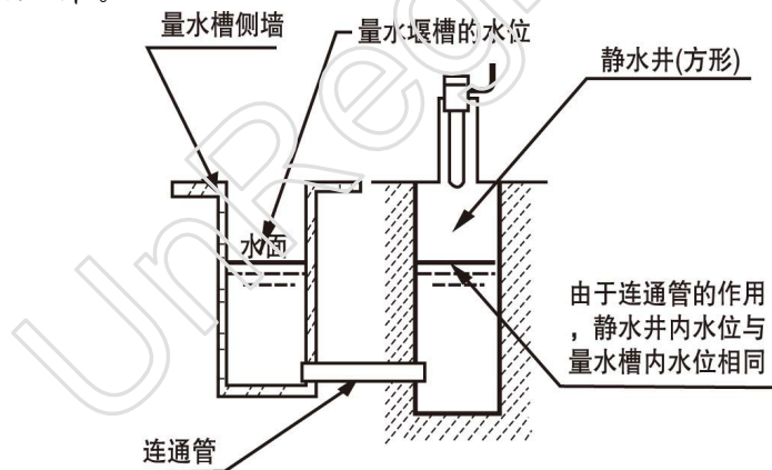
图 4.2.3、静水井安装
