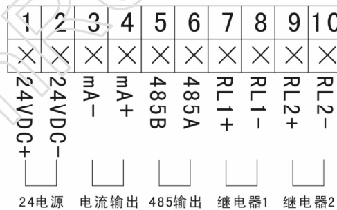
图 4.5.4、一体式明渠流量计 24VDC 接线端子示意图
