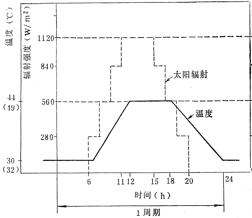
图 1 循环热效应日循环
