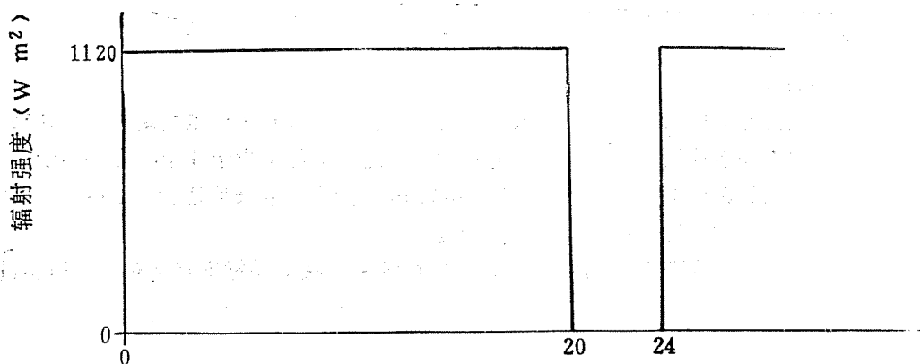
图2 稳态长期光化学效应日循环
