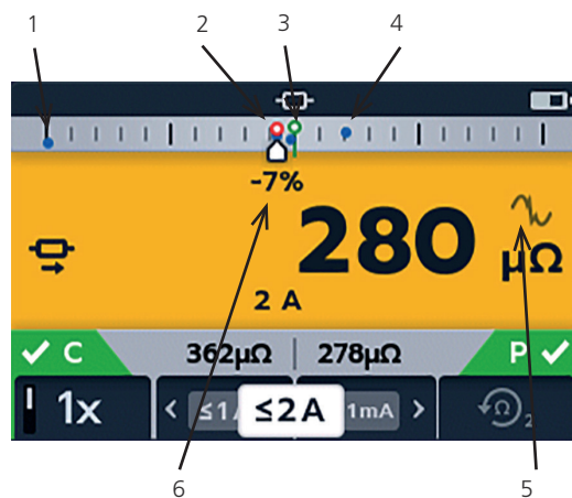
DLRO2 带有差值表的彩色显示屏
