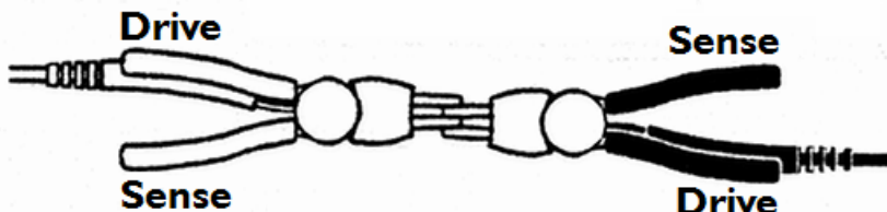
图 3-7 错误的测试端短路方法
