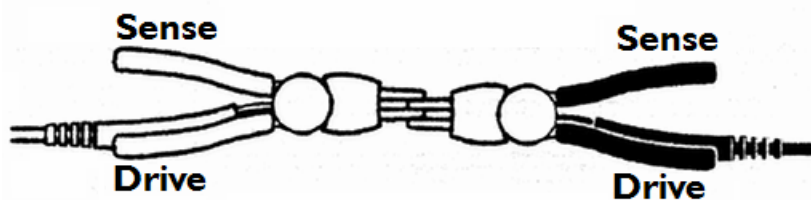
图 3-6 正确的测试端短路方法
