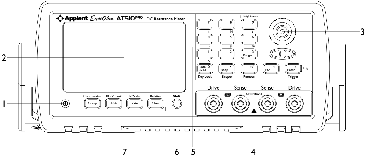
图 3-1 前面板
