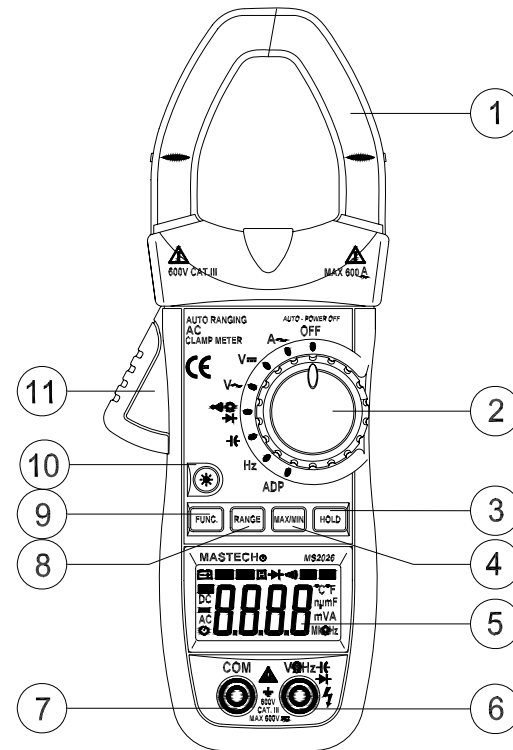
面板示意图
