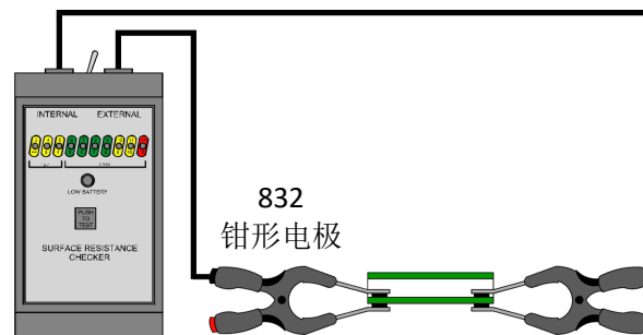
(5) 钳形电极测试示意图
